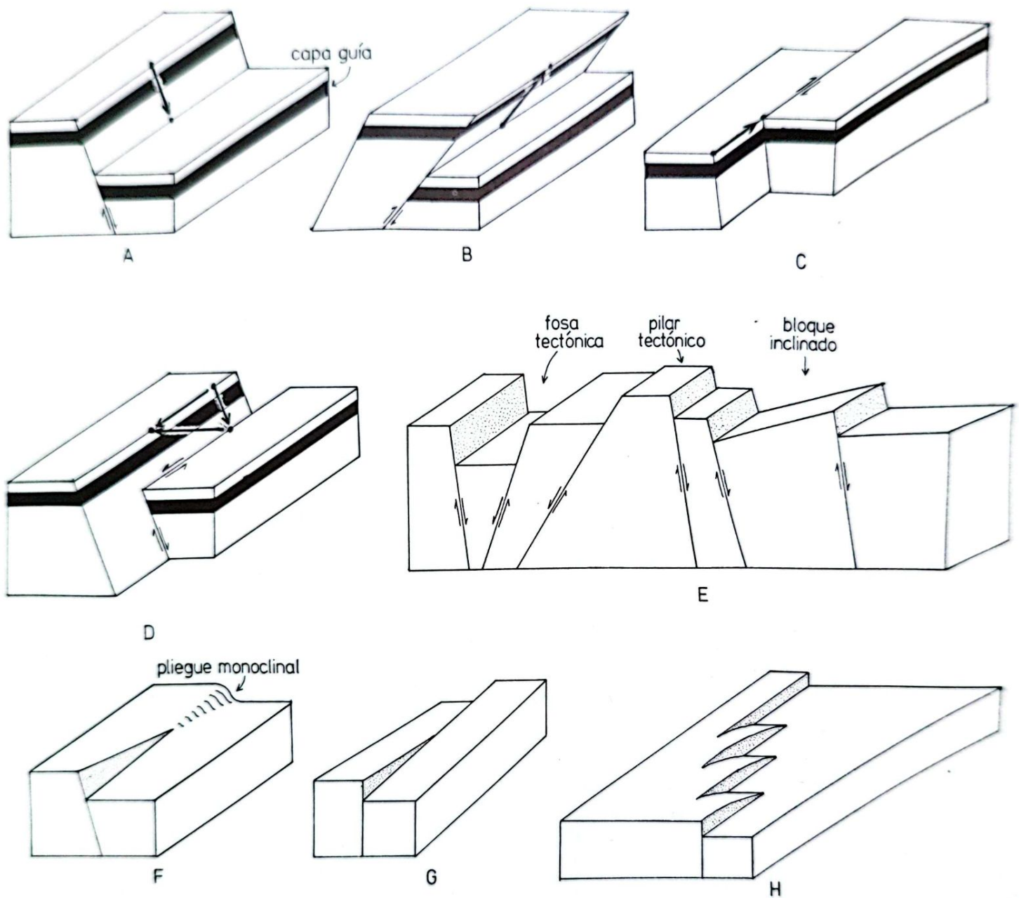
Figura 21. Principales tipos de fallas geológicas, indicadas esquemáticamente como bloques desplazados de la litosfera. El desplazamiento relativo entre los bloques está indicado por la capa guía de color negro. A. Falla normal: desplazamiento vertical hacia abajo. El plano de la falla está inclinado con ángulo alto (buzamiento alto)
