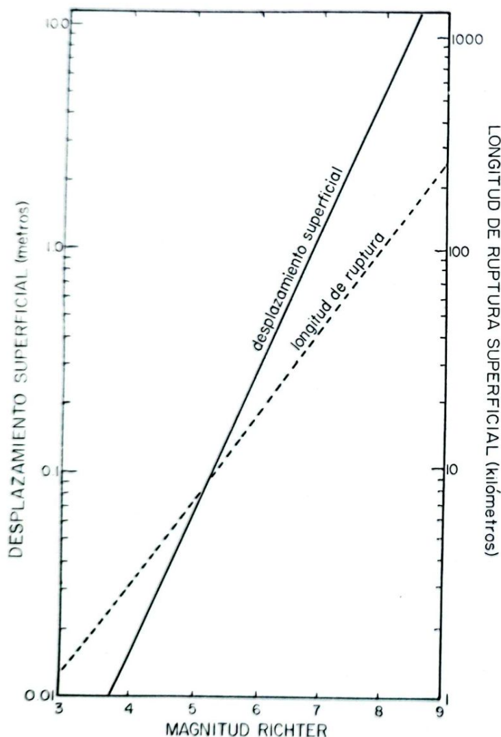
Figura 34. Relación entre la magnitud Richter de un terremoto, el desplazamiento superficial en metros y la longitud total de ruptura superficial en kilómetros, basado en datos de fallas en todo el mundo (simplificado según Bonilla y Buchanan, 1970, y Mark, 1977).
