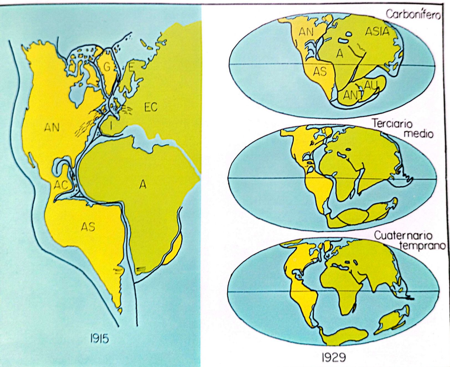
Figura 3. Deriva de los continentes según Wegener en 1915 y 1929. Se muestran reconstrucciones del supercontinente Pangaea para tres periodos geológicos (Tabla 1). Símbolos: A: Africa; AN: América del Norte; AS: América del Sur; E: Escandinavia; ANT: Antártida; AU: Australia; EC: Europa Central; G: Groenlandia.
