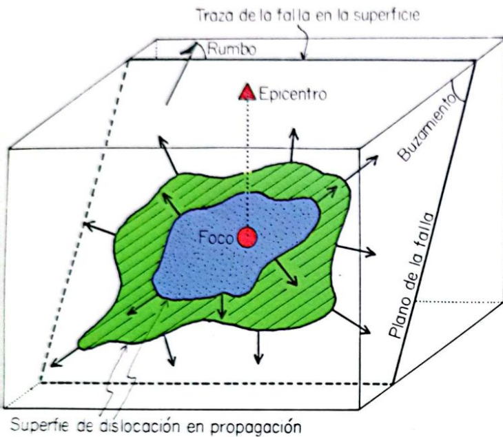
Figura 16. Ilustración esquemática del mecanismo de ruptura a lo largo de una falla geológica (adaptado de Bolt, 1981, Fig. 6). El plano de la falla está definido por su rumbo (ángulo entre la dirección del norte magnético y la traza de la falla en la superficie) y el buzamiento (ángulo entre el plano de la falla y la horizontal). En el foco se produce la dislocación inicial, o ruptura, la cual produce superficies de dislocación que se propagan en todas direcciones sobre el plano de la falla, produciendo, a su vez, las vibraciones características del terremoto.
