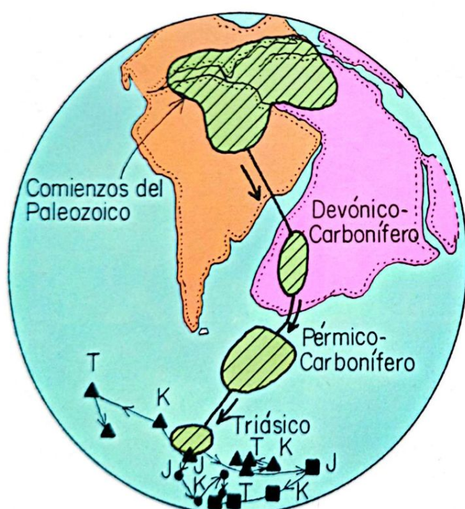
Figura 6. Mapa de los fondos oceánicos mostrando las prominencias oceánicas (línea gruesa) cortadas y desplazadas por fallas (líneas finas) y las fosas marinas (sombreado con rayas) según Heirtzler, 1976. Las regiones sísmicas se denotaron por puntos y la densidad de los puntos representa la frecuencia relativa de los terremotos. Las líneas finas cortadas, simétricas con respecto a las prominencias, representan alineaciones de anomalías magnéticas (ver Fig. 11); los números re-
