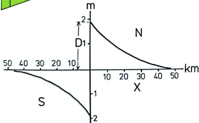
Figura 30. Representación gráfica del desplazamiento, profundidad de ruptura y deformación a lo largo de una falla activa. En el diagrama superior, en la traza superficial se detecta un desplazamiento rumbo-deslizante hacia la derecha, de magnitud D. La profundidad (P) hasta la cual llega la ruptura en el plano de la falla varía de acuerdo con las condiciones locales de la litosfera, pero corresponde a la profundidad a la cual el comportamiento de las rocas, debido a la presión y temperatura, pasa de elástico (sólido) a dúctil o plástico. Las líneas en el diagrama tridimensional representan el campo de deformación en la litosfera. El gráfico inferior muestra el desplazamiento medido en metros a distancias progresivamente mayores (X; en kilómetros) desde la traza superficial de la falla en los dos bloques adyacentes a la falla (N y S).
