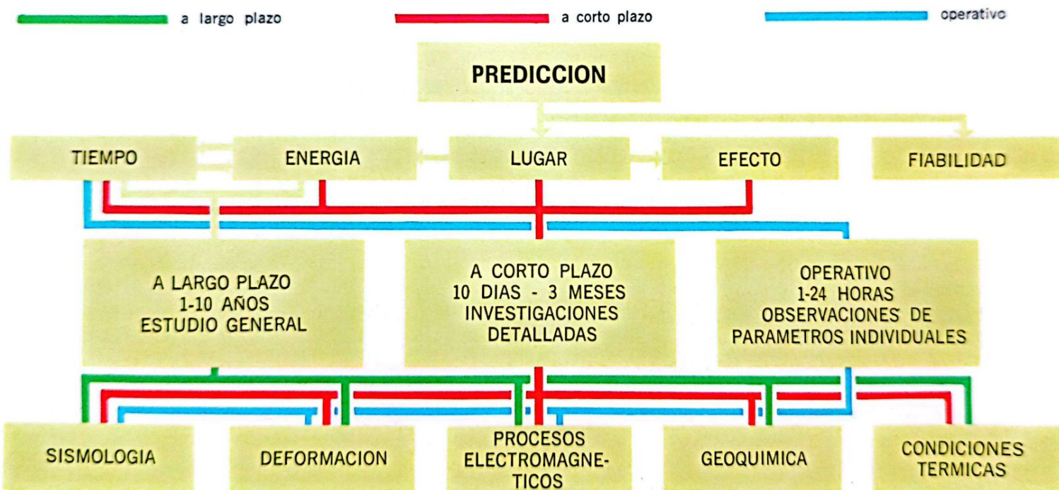
Figura 31. Factores que intervienen en la predicción sísmica (simplificado según Savarenskij y Nersesov, 1980). Ver el texto para la explicación detallada.
