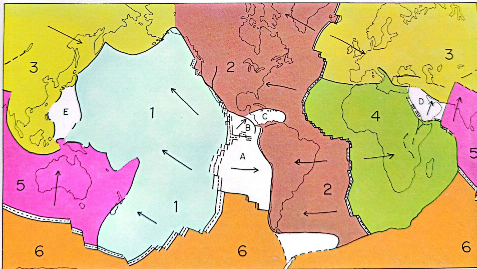
Figura 13. Mapa mostrando las seis placas principales de la litosfera, según Bullard (1969) (1: Pacífico; 2: América; 3: Eurasia; 4: África; 5: Índico; 6: Antártida). Existen también varias placas menores (A: de Nazca; B: del Caribe; C: del Caribe; D: Árabe; E: del Japón). Las flechas indican el movimiento relativo de las placas.
