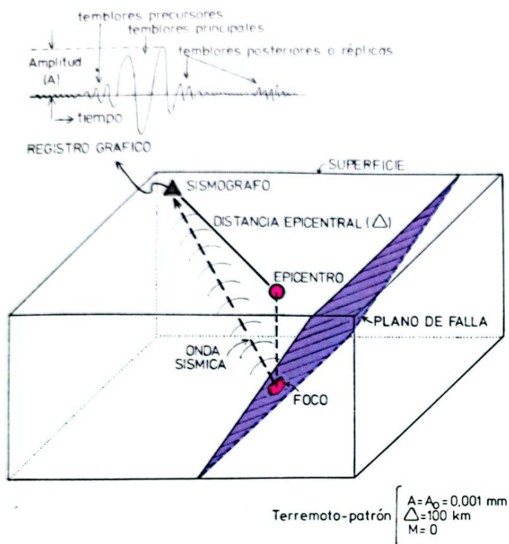
Figura 20. Ilustración esquemática de la detección de un terremoto. Al producirse la ruptura en alguna parte de un plano de falla, se generan ondas sísmicas las cuales se desplazan a través del material de la litosfera. El sitio de la ruptura se denomina el foco del terremoto. El sitio donde la línea que conecta el foco con el centro de la Tierra aflora en la superficie, se denomina epicentro. La detección de las ondas sísmicas se realiza en un sismógrafo colocado a una distancia cualquiera del terremoto (distancia epicentral, \Delta ). En el sismógrafo, estas ondas sísmicas generan un gráfico en el cual aparecen las vibraciones correspondientes a las ondas. La amplitud ( A ) es la distancia entre la línea central del gráfico (o sismograma) y la anchura de cada onda. La amplitud define en forma gráfica la magnitud ( M ) de un terremoto. Según Richter (1958) la magnitud 0 corres-
