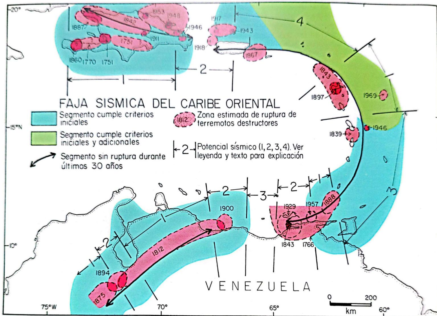
Figura 36. La faja sísmica del Caribe Oriental definida por los terremotos destructores más importantes de la región (simplificado y modificado según Kelleher y otros, 1973, y Nishenko y McCann, 1981). Los segmentos de esta faja indicados en color azul cumplen con los criterios iniciales de Kelleher y otros (1973): son parte de un borde entre dos placas, con desplazamientos rumbo-deslizantes (norte y sur) o inverso o de corrimiento (este), y no han sufrido ruptura durante los últimos 30 años. El segmento de la faja sísmica indicado en color verde cumple con estos criterios y, además, con por lo menos uno de los criterios adicionales: un registro histórico de uno o más terremotos grandes, indicios de que el intervalo de retorno para terremotos grandes es similar al intervalo transcurrido desde el último terremoto, y que en el segmento puede producirse el próximo evento sísmico. La zona de ruptura para terremotos destructores individuales (color rojo) fue estimada con base en los efectos descritos en publica-
