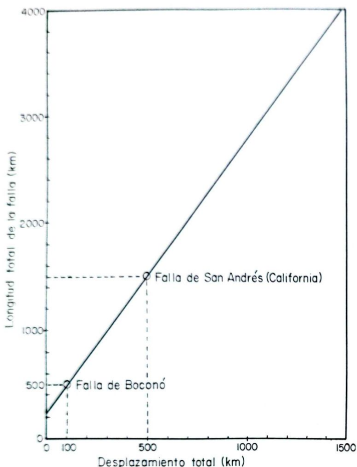
Figura 29. Representación gráfica de la relación entre la longitud de una falla rumbo-deslizante y el desplazamiento total a través de ella, según compilación mundial de 15 fallas con datos confiables, realizada por H. W. Menard (1962). En el cálculo estadístico de esta relación se incluyeron los datos de la falla de Boconó (500 km. de longitud total y aproximadamente 100 km. de desplazamiento rumbo-deslizante hacia la derecha total). Si se considera la longitud total del sistema de fallas de Boconó-Morón-El Pilar (más de 1.300 km.), según esta relación, el desplazamiento total a lo largo del sistema debería ser más de 400 km., en sentido rumbo-deslizante hacia la derecha. El hecho de que, hasta el presente, no
